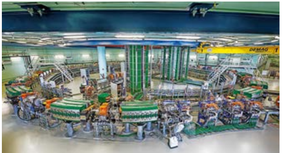
Nur sechs Mal weltweit, ein Mal in Wiener Neustadt: ein Synchrotron-basierter Teilchenbeschleuniger, der verschiedene Partikel für Therapie und Forschung bereitstellt.
